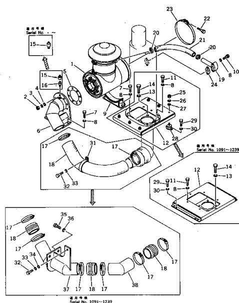
Fig. 104 エアー クリーナ および パイピング (適用 機種 Serial No. 1005~1239)
