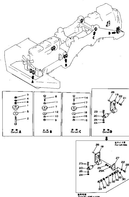
エンジン トルク コンバータ および トランスミッション マウンティング Fig. 103 ENGINE TORQUE CONVERTER AND TRANSMISSION MOUNTING (適用号機 Serial No. 1005~1239)
