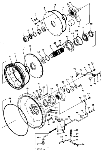
Fig. 101 アウトプットシャフト (適用機種) OUT PUT SHAFT (Serial No. 1005~1239)
