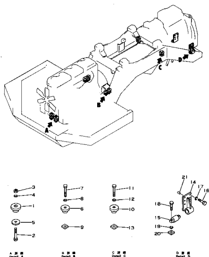
エンジン トルク コンバータ および トランスミッション マウンティング Fig. 103A ENGINE TORQUE CONVERTER AND TRANSMISSION MOUNTING (適用 号機 Serial No. 1240~)
