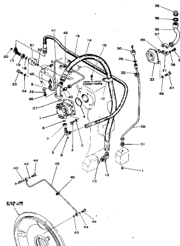
PTO A-ブオイルパイピング (適用機種) Fig. 103 PTO LUB. OIL PIPING (Serial No. 1008--1083)
