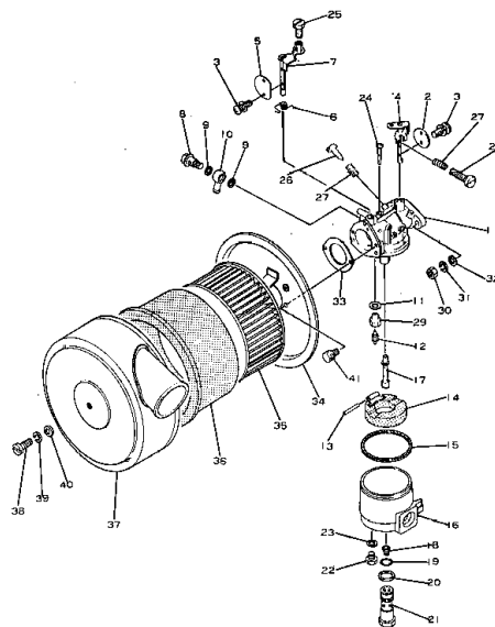
キャブレタ および エアー クリーナ Fig. 106 A CARBURETOR AND AIR CLEANER (適用機種 Serial No. 2501~)
