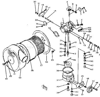
キャブレタ および エアークリーナ Fig. 106 CARBURETOR AND AIR CLEANER (適用号機 Serial No. 1003~2500)
