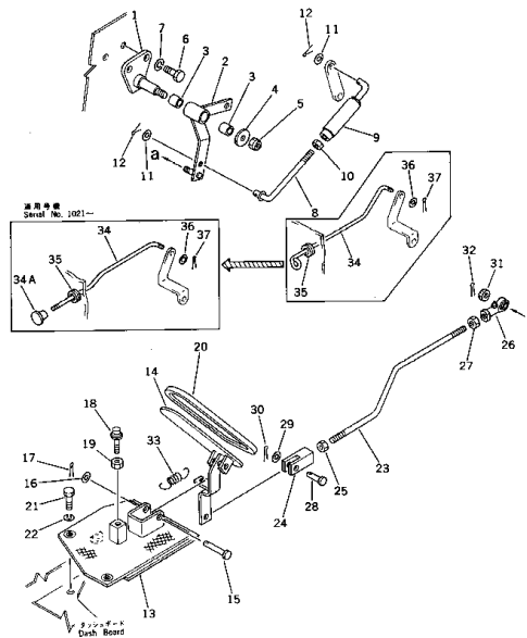
アクセル ペダル および エンジン ストップ レバー Fig. 122 ACCELERATOR PEDAL AND ENGINE STOP LEVER
