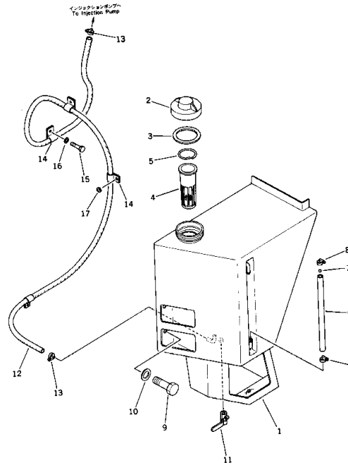
Fig. 141 FUEL TANK フュエルタンク
