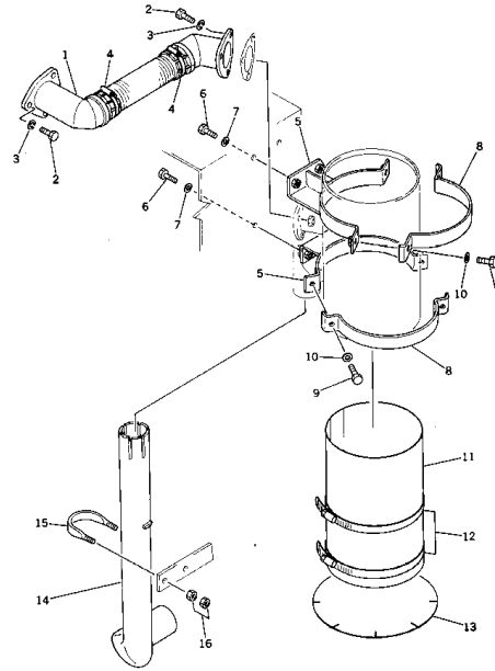
エキゾーストコネクションおよびマフラー Fig. 117 EXHAUST CONNECTION AND MUFFLER
