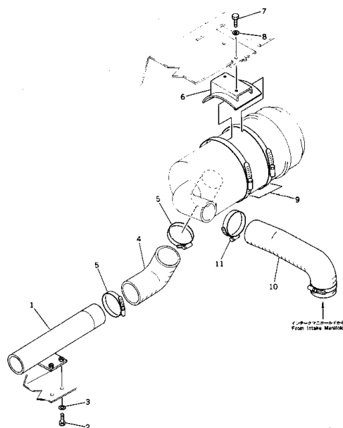
エアークリーナ コネクション Fig. 115 AIR CLEANER CONNECTION
