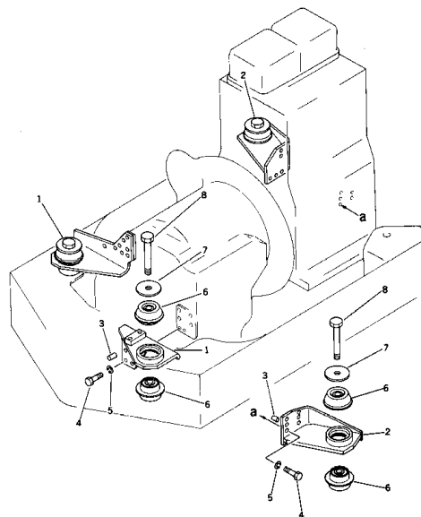
エンジン および トランスミッション 取付 図 Fig.101 ENGINE AND TRANSMISSION MOUNTING PARTS
