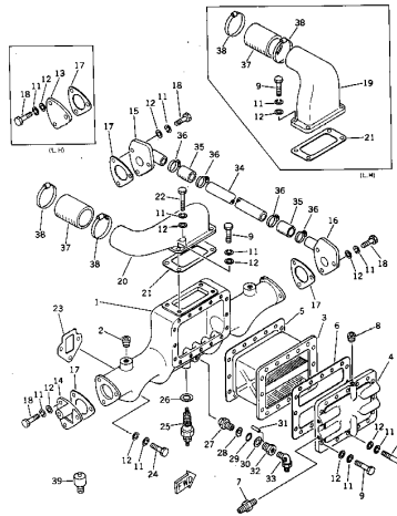
Fig. 111 エアークラウド マニホールド および 接続 AIR INTAKE MANIFOLD AND CONNECTION (Engine No. 430077-535023)
