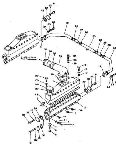
Fig. 111 エアー インテーク マニホールド および コネクション AIR INTAKE MANIFOLD AND CONNECTION
