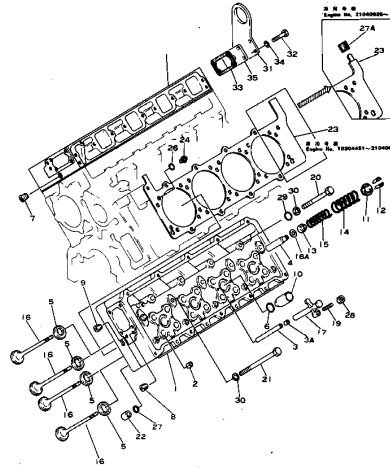
シリンダ ヘッド Fig. 101 CYLINDER HEAD
