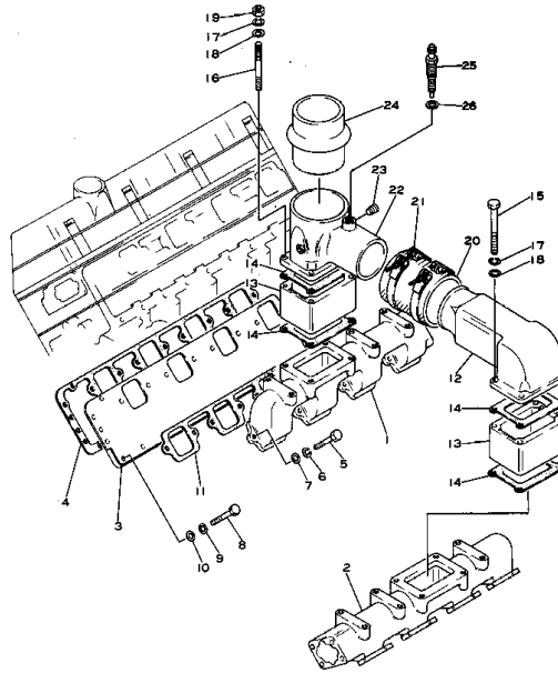
エアインテークマニホールド および コネクション Fig. 104 AIR INTAKE MANIFOLD AND CONNECTION
