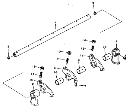
Fig.103 ロックレバーおよびシャフト ROCKER LEVER AND SHAFT
