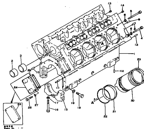
Fig.201 シリンダブロック CYLINDER BLOCK
