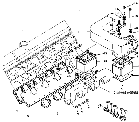
Fig.104 エアー インテーク マニホールド AIR INTAKE MANIFOLD
