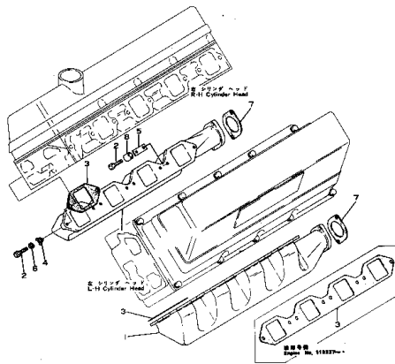
Fig.105 エキゾースト マニホールド EXHAUST MANIFOLD
