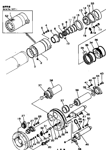
パイロットヘッド Fig. 112 PILOT HEAD (2/4) ( Swing Jack and Potentiometer )
