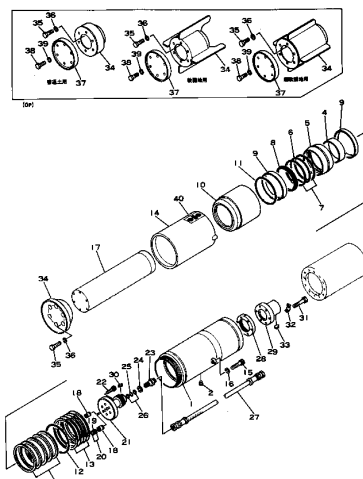
パイロットヘッド (ヘッドおよびパイロットジャック) Fig. 111 PILOT HEAD (1/4) (Head and Pilot Jack) (適用機種 Serial No. 1005~1076)
