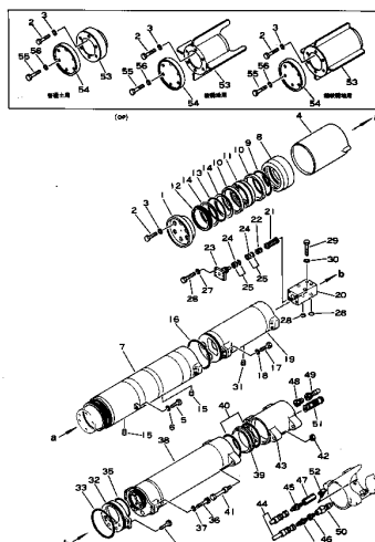
パイロットヘッド (ヘッドおよびボディ) (適用機種) Fig. 101 PILOT HEAD (Head and Body) (Serial No. 1005~1076)
