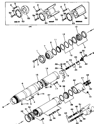
パイロットヘッド (ヘッドおよびボデー) (通称等価) Fig. 101A PILOT HEAD (Head and Body) (Serial No. 1077~)
