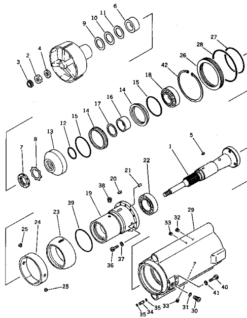
パイロットヘッド Fig. 102 PILOT HEAD (2/7)
