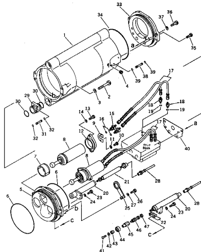
パイロットヘッド Fig. 105 PILOT HEAD (5/7)
