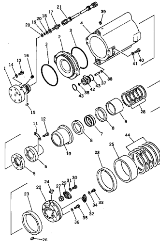
パイロットヘッド Fig. 104 PILOT HEAD (4/7)
