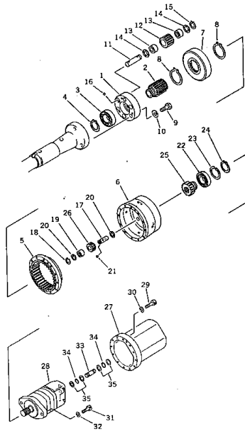
パイロットヘッド Fig. 103 PILOT HEAD (3/7)
