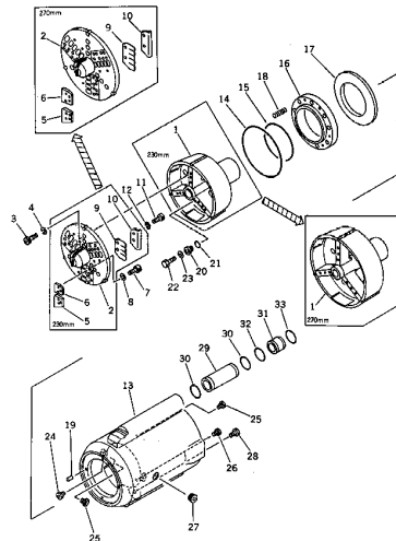
パイロットヘッド Fig. 101 PILOT HEAD (1/7)
