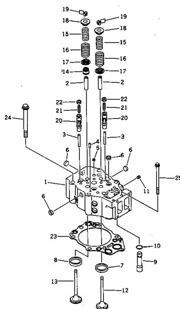
シリンダ ヘッド FIG. 1001 CYLINDER HEAD
