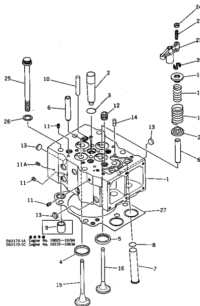
FIG. 101 シリンダヘッド CYLINDER HEAD
