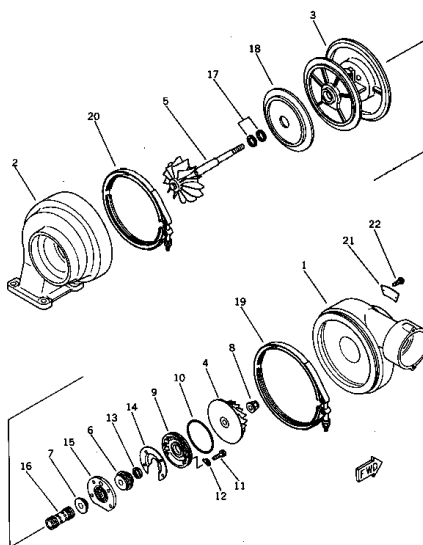
ターボチャージャー FIG. 141 TURBOCHARGER
