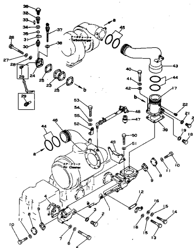
FIG. 1113 エア- インテーク マニホールド および コネクション 適用 機種 適用 年 月 日 AIR INTAKE MANIFOLD AND CONNECTION (ENGINE NO. 22146 - 28769)
