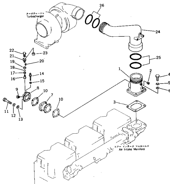
FIG. 1311 エアインテークコネクション AIR INTAKE CONNECTION
