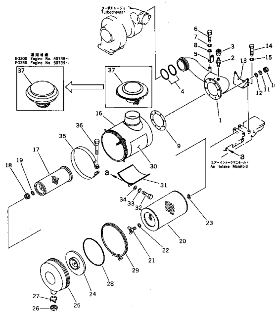
エアークリーナ FIG. 1401 AIR CLEANER (EG300, 350)
