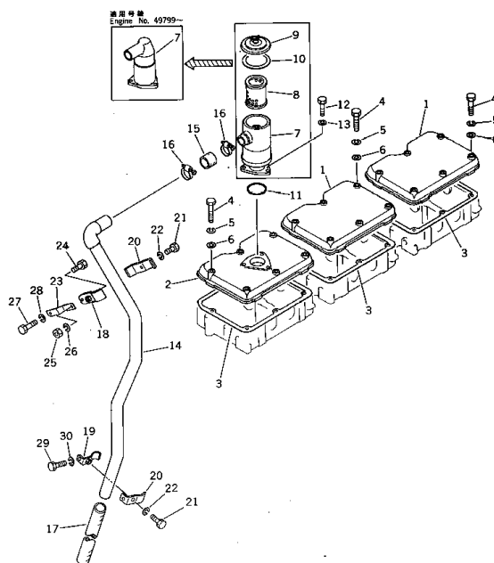
FIG. 1151 ロッカーアームハウジングカバー ROCKER ARM HOUSING COVER
