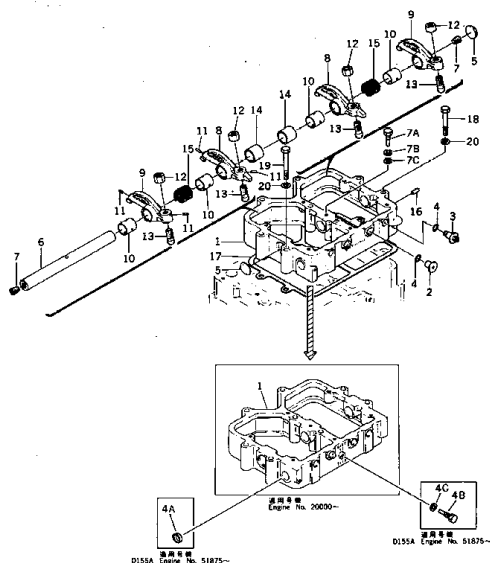
ロ ッ カ アームおよび ハウジング FIG. 1103 ROCKER ARM AND HOUSING
