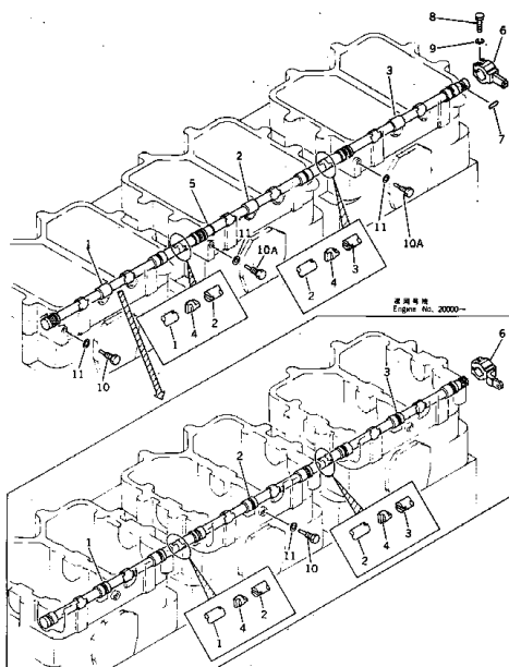
コンプレッション リリース FIG. 1107. COMPRESSION RELEASE
