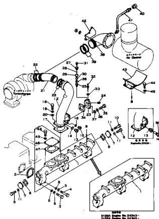
エアークリーナースキームおよびコネクشن FIG. 1112A AIR INTAKE MANIFOLD AND CONNECTION 適用機種 (S6D155-4A ENGINE NO. 20000 - 40560) (S6D155-4B ENGINE NO. 20000 - 40560)
