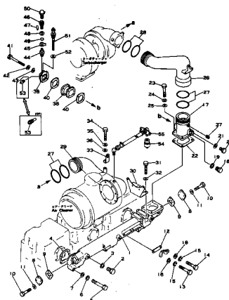
エア-インテークマニホールド及び コネクション FIG. 1112 AIR INTAKE MANIFOLD AND CONNECTION 適用機 (S6D155-4A ENGINE NO. 10014 - 19999) (S6D155-4B ENGINE NO. 10016 - 19999)
