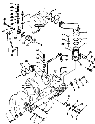
エア-インテークマニホールド及び コネクション FIG. 1112 AIR INTAKE MANIFOLD AND CONNECTION 適用機 (S6D155-4A ENGINE NO. 10014 - 19999) (S6D155-4B ENGINE NO. 10018 - 19999)
