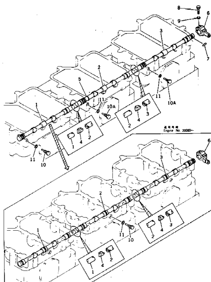
コンプレッションリリース FIG. 1111 COMPRESSION RELEASE
