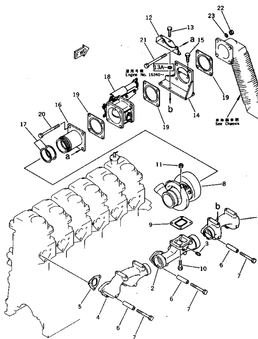
エキゾースト マニホールド および ターボチャージャ FIG. 1501 EXHAUST MANIFOLD AND TURBOCHARGER
