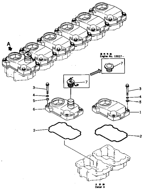
ロッカー アーム ハウジング カバー FIG. 1151 ROCKER ARM HOUSING COVER
