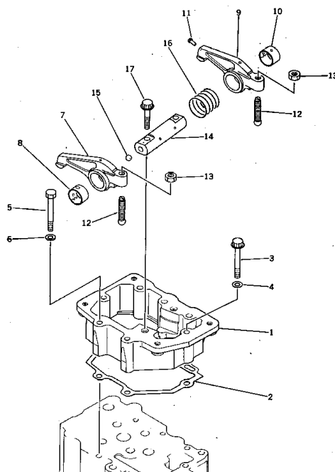
ロッカ アーム および ハウジング FIG. 1101 ROCKER ARM AND HOUSING
