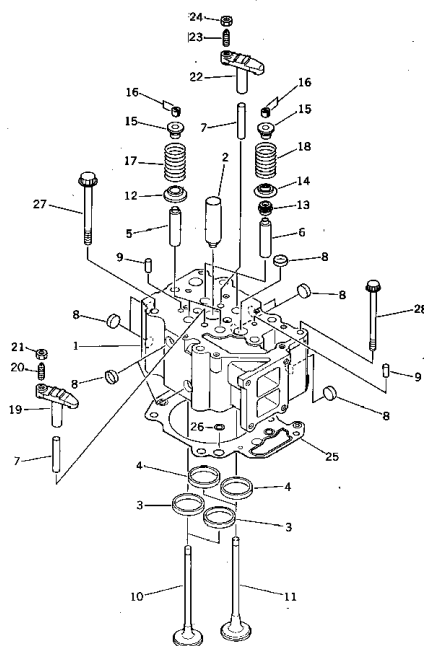
シリンダ ヘッド FIG. 1001 CYLINDER HEAD
