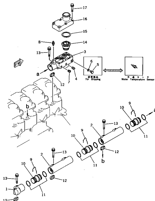
ウォーター マニホールド および サーモスタット FIG. 1701 WATER MANIFOLD AND THERMOSTAT
