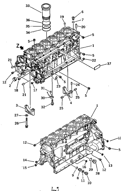
シリンダ ブロック FIG. 2001 CYLINDER BLOCK
