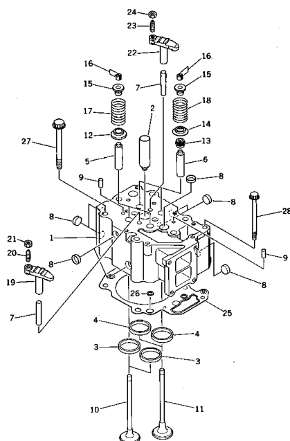
シリンダ ヘッド 適用号機 FIG. 1001 CYLINDER HEAD (ENGINE NO. 19950-26563)
