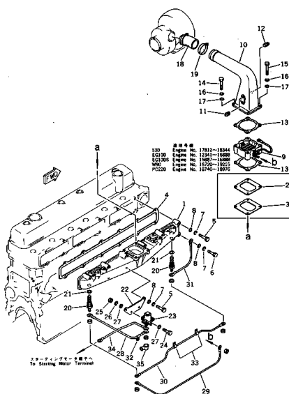
エア インテーク マニホールド 適用機種 FIG. 111A AIR INTAKE MANIFOLD (EG100 ENGINE NO. 12341-) (EG100S ENGINE NO. 15887-)
