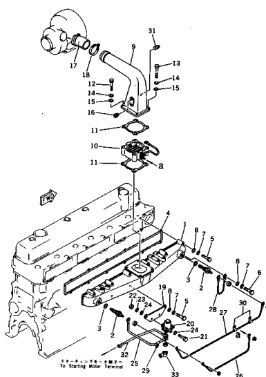
エア インテーク マニホールド 適用機種 FIG. 111 AIR INTAKE MANIFOLD (EG100 ENGINE NO. 11370-12340) (EG100S ENGINE NO. 11462-15886)
