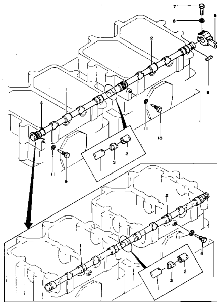
コンプレッション リリース Fig. 107 COMPRESSION RELEASE
