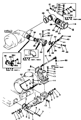
エアークリーナー マニホールド および コネクション Fig. 111 AIR INTAKE MANIFOLD AND CONNECTION
