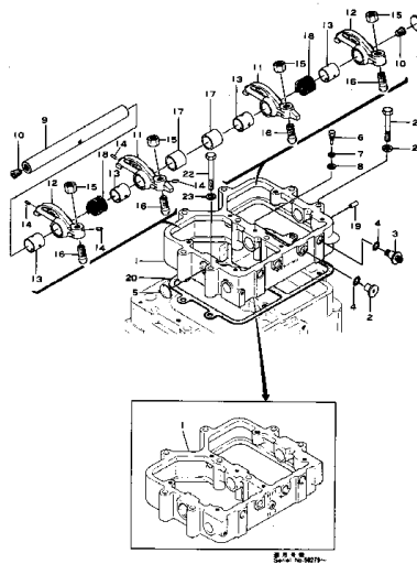
ロッカ アーム および ハウジング Fig.103 ROCKER ARM AND HOUSING
