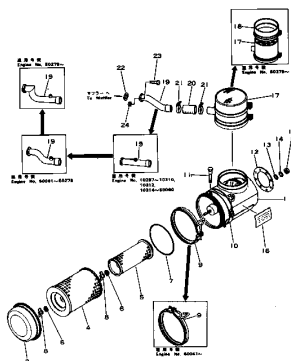
エアークリーナ および プリクリーナ Fig.115 AIR CLEANER AND PRECLEANER
