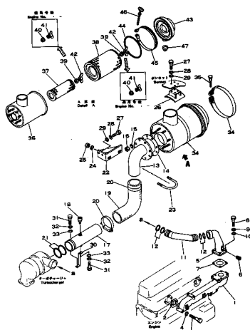
エア インテーク マニホールド 及び エア クリーナ FIG. 115 AIR INTAKE MANIFOLD AND AIR CLEANER (S4D120-11D ENGINE NO. 90126- )
