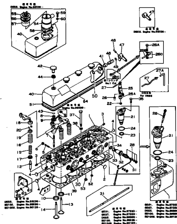
シリンダ ヘッド、カバー、および プリコンバッション チャンバ FIG. 101 CYLINDER HEAD, COVER AND PRECOMBUSTION CHAMBER
