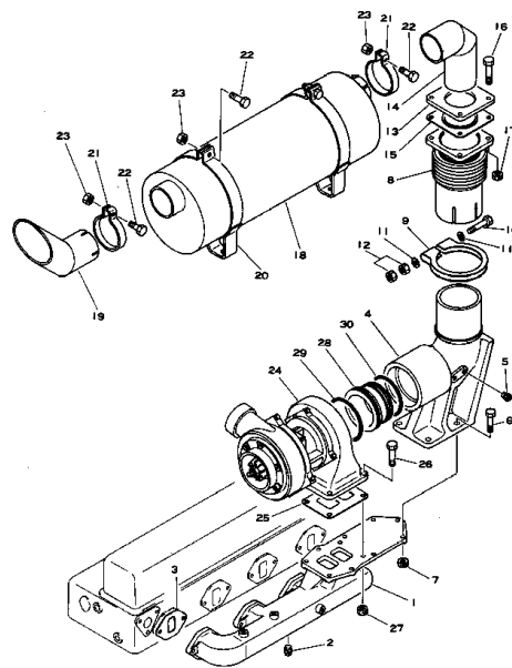
エキゾースト マニホールド および マフラー FIG. 124 EXHAUST MANIFOLD AND MUFFLER 適用機種 (S4D120-11C ENGINE NO. 89595-)
