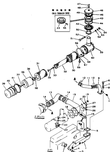
エアークリーナとエアークリーナホルダおよびエアークリーナ 適用車種 FIG. 111A AIR INTAKE MANIFOLD AND AIR CLEANER (ENGINE NO. 75212-)
