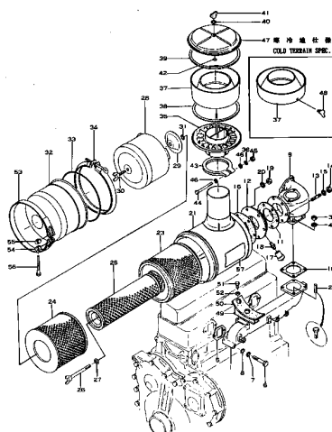
エアークリーナマニホールド および エアークリーナ 適用 機種 FIG. 111 AIR INTAKE MANIFOLD AND AIR CLEANER (ENGINE NO. 50025 ~ 75211)
