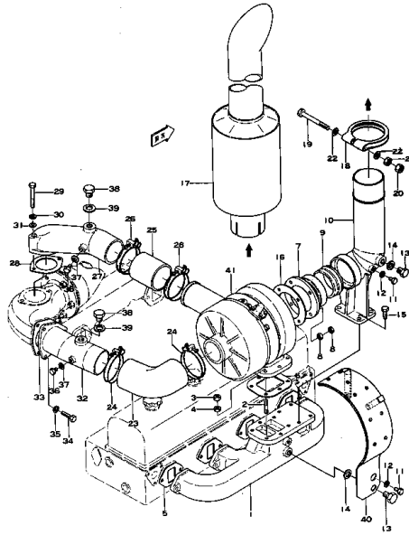
エキゾーストマニホールドおよびマフラー 適用機種 FIG. 121 EXHAUST MANIFOLD AND MUFFLER (ENGINE NO. 50025 - 56382)
