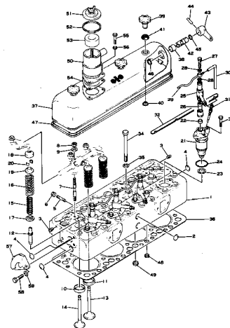
シリンダ ヘッド、カバー 組み プリコンバッション チャンバ FIG. 102 CYLINDER HEAD, COVER AND PRECOMBUSTION CHAMBER
