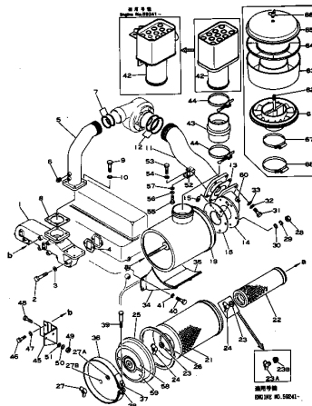
エアー インテーク マニホールド および エアー クリーナ FIG. 112 AIR INTAKE MANIFOLD AND AIR CLEANER 図 112 (S4D120-11B ENGINE NO. 85088-)
