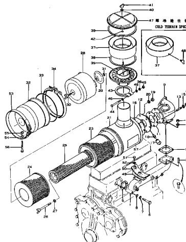
エアークリーナースキームおよびエアークリーナースキーム FIG. 111 AIR INTAKE MANIFOLD AND AIR CLEANER (ENGINE NO. 50026-75211)
