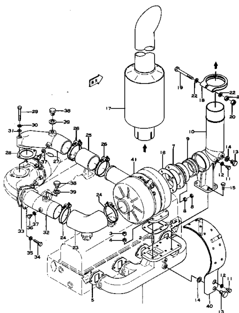
エキゾーストマニホールドおよびマフラー 図用番線 FIG. 121 EXHAUST MANIFOLD AND MUFFLER (ENGINE NO. 50026 - 54936)
