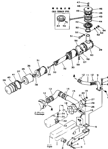
エアークリーナとエアークリーナホルダ及びエアークリーナ FIG. 111A AIR INTAKE MANIFOLD AND AIR CLEANER (ENGINE NO. 75212 -)
