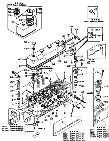
シリンダヘッド・カバーおよび予燃焼室 FIG. 101 CYLINDER HEAD, COVER AND PRECOMBUSTION CHAMBER
