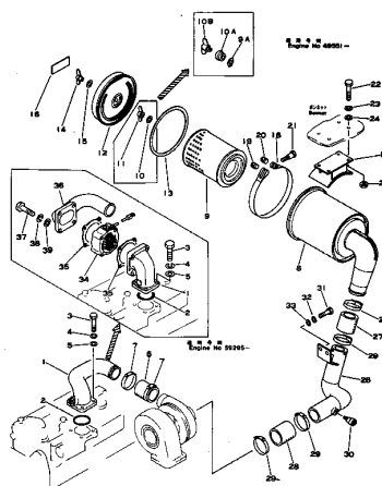
エア- インテーク コネクション 及び エア- クリーナ FIG. 1115 AIR INTAKE CONNECTION AND AIR CLEANER 適用機種 (EGSS ENGINE NO. 44605- )
