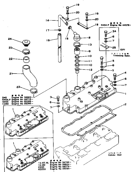
シリンダヘッドカバー FIG. 1105 CYLINDER HEAD COVER
