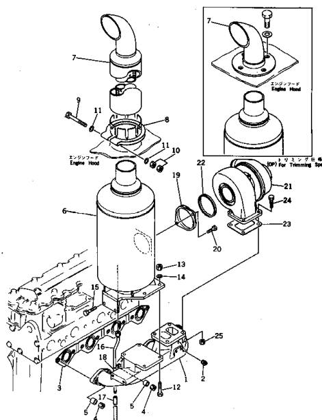
エキゾースト マニホールド および マフラー FIG. 1121 EXHAUST MANIFOLD AND MUFFLER
