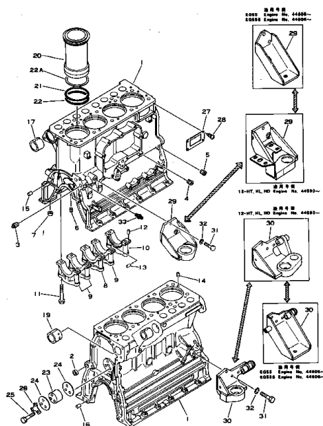
シリンダー ブロック FIG. 1201 CYLINDER BLOCK
