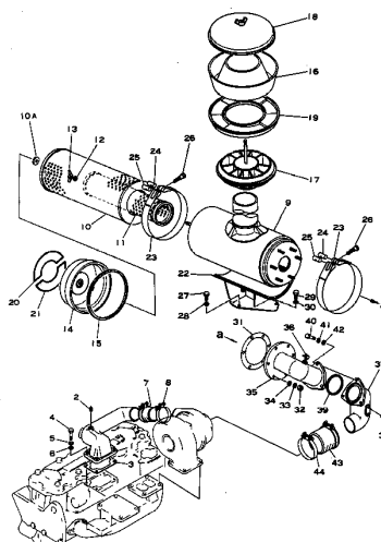
エア- インテーク コネクション および エア- クリーナ FIG. 113 AIR INTAKE CONNECTION AND AIR CLEANER
