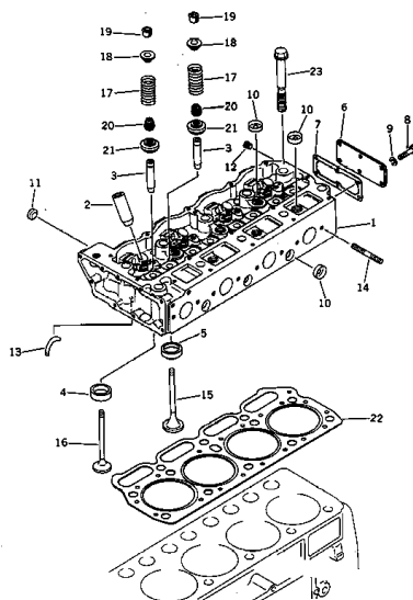
FIG. 101 シリンダヘッド CYLINDER HEAD
