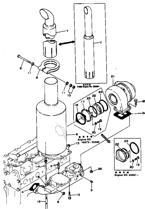
エキゾースト マニホールド および マフラー FIG. 123 EXHAUST MANIFOLD AND MUFFLER
