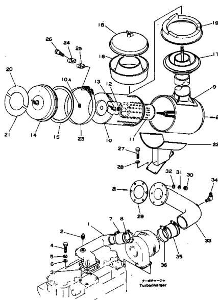
エア インテーク コネクション 及び エア クリーナ FIG. 114 AIR INTAKE CONNECTION AND AIR CLEANER
