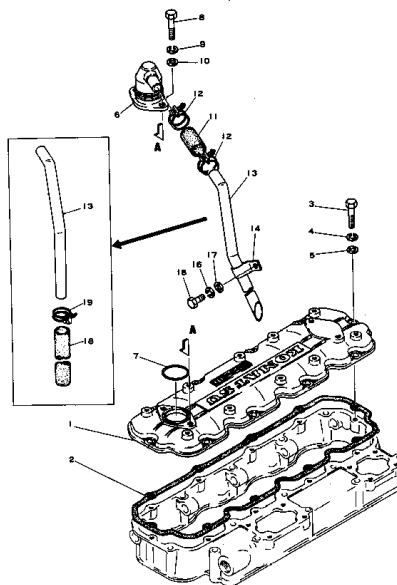
シリンダ ヘッド カバー FIG. 105 CYLINDER HEAD COVER
