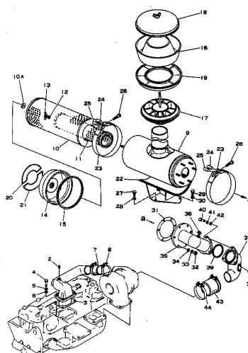
エアークリーナ コネクション 及び エアークリーナ FIG. 113 AIR INTAKE CONNECTION AND AIR CLEANER
