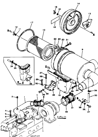
エアークリーナ マニホールド組立図 FIG. 112 AIR INTAKE MANIFOLD AND AIR CLEANER
