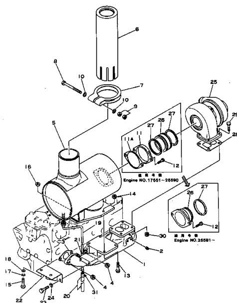
エキゾースト マニホールド および マフラー FIG. 122 EXHAUST MANIFOLD AND MUFFLER
