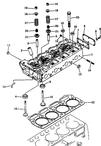
FIG. 101 シリンダヘッド CYLINDER HEAD
