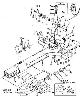
Fig. 103 DRAWBAR (Serial No. 1001-...)
