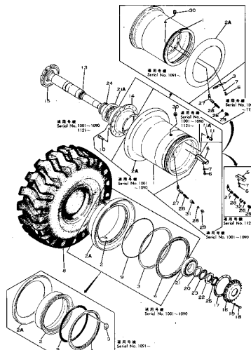
リヤアサスル および ホイール (機 用 車 用) Fig. 102 REAR AXLE AND WHEEL (Serial No. 1001-...)
