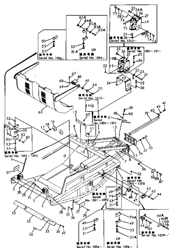
ボウルおよびエプロン (適用機種) (Serial No. 1001~)
