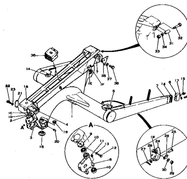
Fig. 105 YOKE (適用機種 Serial No. 1001~)
