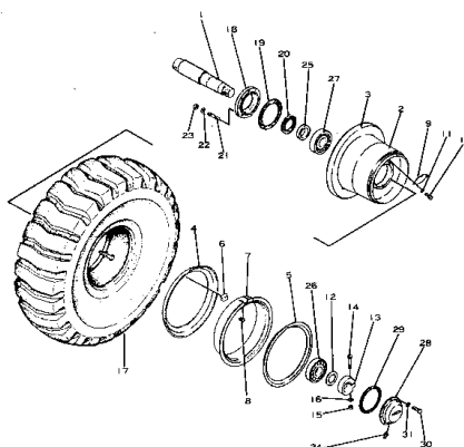
フロント アクスル および ホイール (適用号機) Fig. 101 FRONT AXLE AND WHEEL (Serial No. 1001~)
