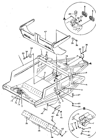
Fig. 104 BOWL AND APRON (適用機種 (適用号機) Serial No. 1001~)
