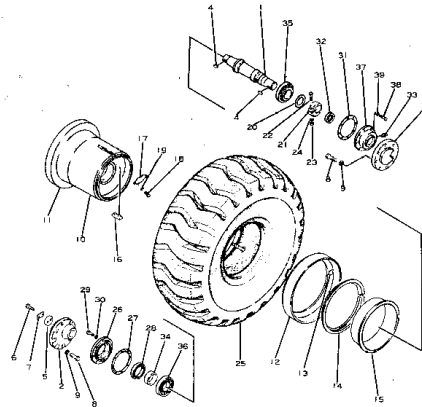
リヤアックス および ホイール (適用機種: Serial No. 1001~) Fig. 102 REAR AXLE AND WHEEL
