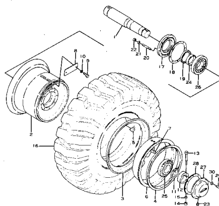
フロント アクセル および ホイール (適用 号 機) F i g. 1 0 1 FRONT AXLE AND WHEEL (Serial No. 1201~)
