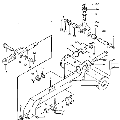
Fig. 103 DRAWBAR (適用号機 Serial No. 1201~)
