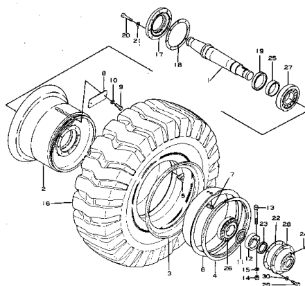
リヤ アクスル および ホイール (適用 号 数) Fig. 1-0 2 REAR AXLE AND WHEEL (Serial No. 1201~)
