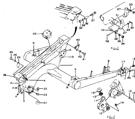
Fig. 105 YOKE (Serial No. 1201~)
