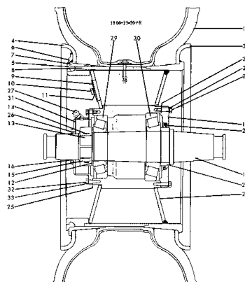
リヤアキス Fig. 102 REAR AXLE
