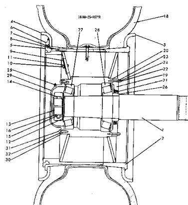
Fig. 101 フロント アクス FRONT AXLE
