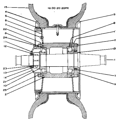
リヤ アクスル および ホイール (適用機種) Fig. 102 REAR AXLE AND WHEEL (Serial No. 1001 ~ 1994)
