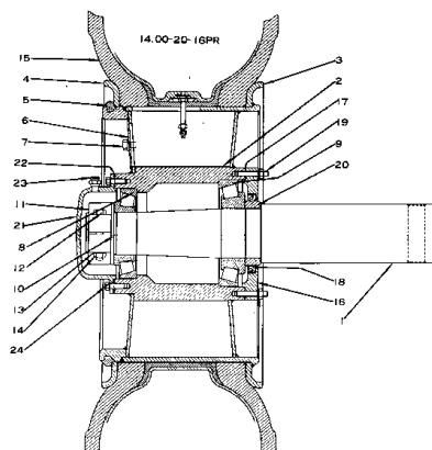
フロント アクセル および ホイール (適用号 表) Fig. 101 FRONT AXLE AND WHEEL (Serial No. 1001 ~ 1994)
