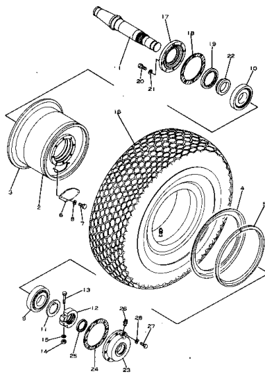
リヤ アクスル およびホイール (適用号機) Fig. 102A REAR AXLE AND WHEEL (Serial No.1995~)
