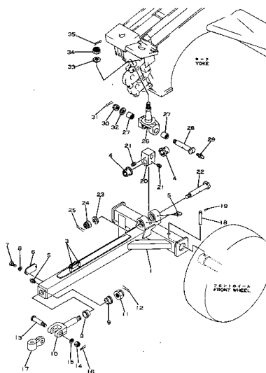
トローバ (適用号機) Fig. 103A DRAWBAR (Serial No. 1995~)
