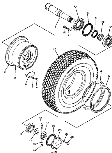
フロント アクスル およびホイール (適用機種 Fig. 101A FRONT AXLE AND WHEEL (Serial No.1995~)
