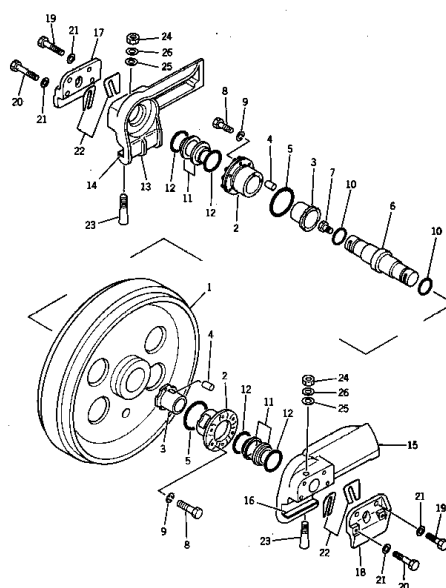
フロントアイドラ Fig. 1115 FRONT IDLER
