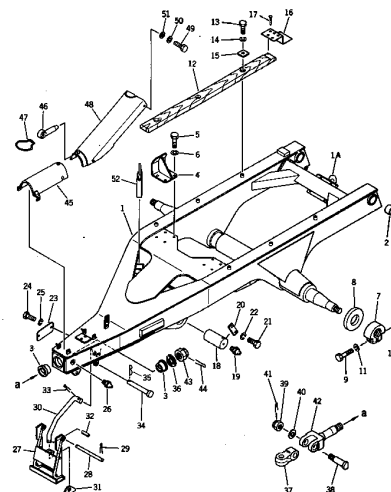
トレーラ フレーム Fig. 1101 TRAILER FRAME
