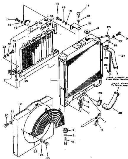
ラジエータおよびオイルクーラ Fig. 131 RADIATOR AND OIL COOLER (適用機種 PW60 Serial No. 1501~1528 PW60N Serial No. 1501~1528)
