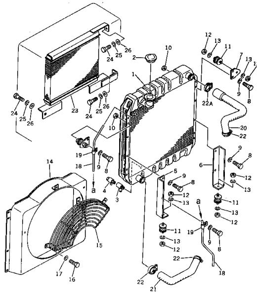
ラジエータ および オイル ク ー ラ Fig. 131A RADIATOR AND OIL COOLER 適用機種 (PW60 Serial No. 1529~) (PW60N Serial No. 1529~)
