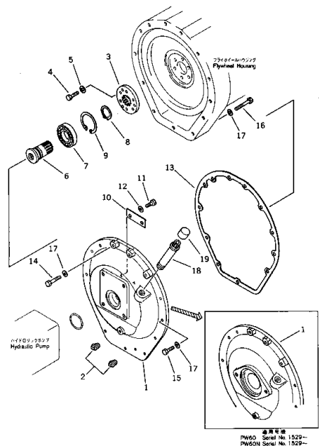
パワー テイク オフ Fig. 105 POWER TAKE OFF
