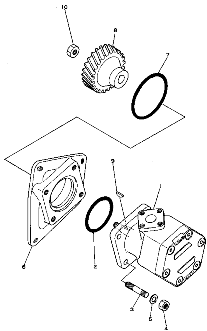
パワータイクオフ (ステアリングポンプ用) Fig. 106 POWER TAKE OFF (For Steering Pump)
