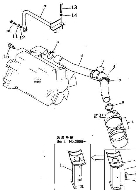
FIG. 1101 エアークリーナ コネクション AIR CLEANER CONNECTION
