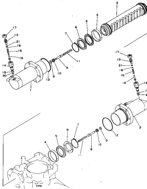
Fig. 211 スイング シリンダ SWING CYLINDER
