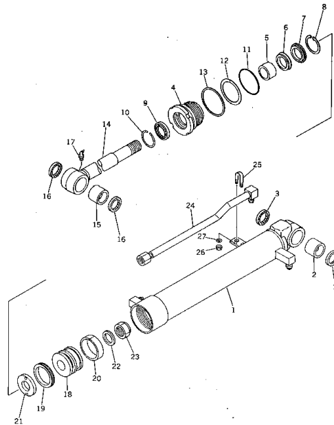
Fig. 141 バケット シリンダ BUCKET CYLINDER
