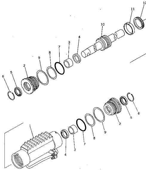
Fig. 211 スイング シリンダ SWING CYLINDER
