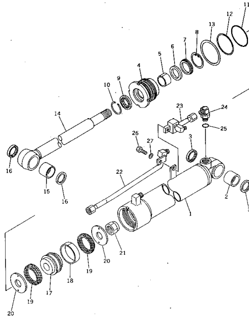
Fig. 121 ブーム シリンダ BOOM CYLINDER
