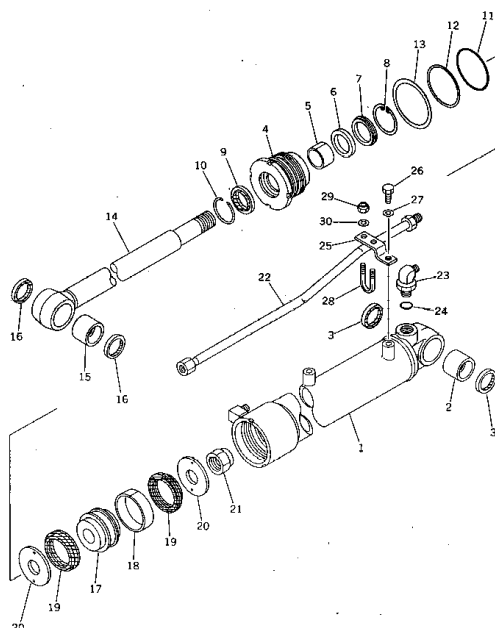
Fig. 131 アーム シリンダ ARM CYLINDER
