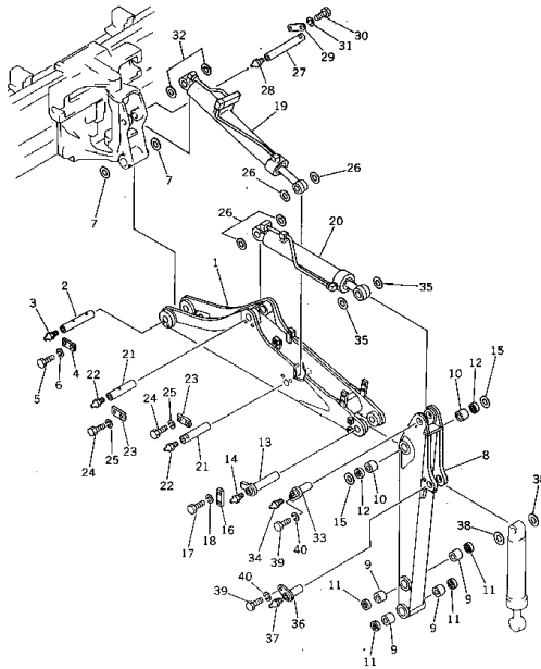
Fig. 101 ブーム および アーム BOOM AND ARM
