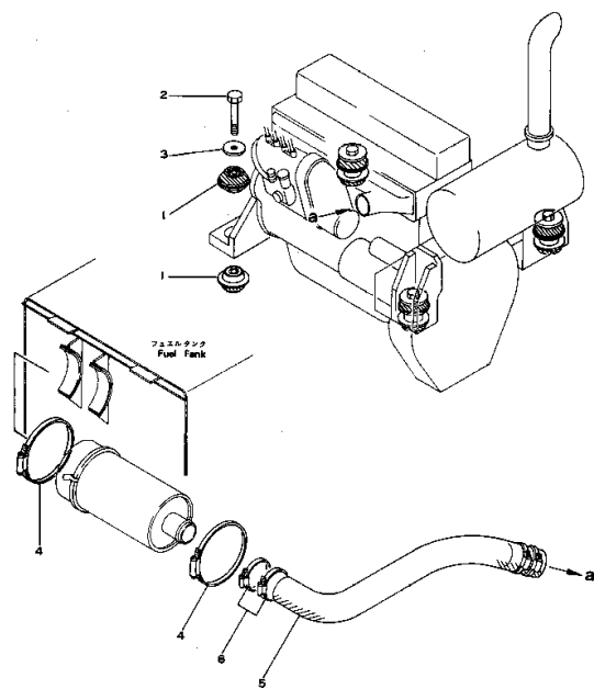
エンジンマウント Fig. 101 ENGINE MOUNT
