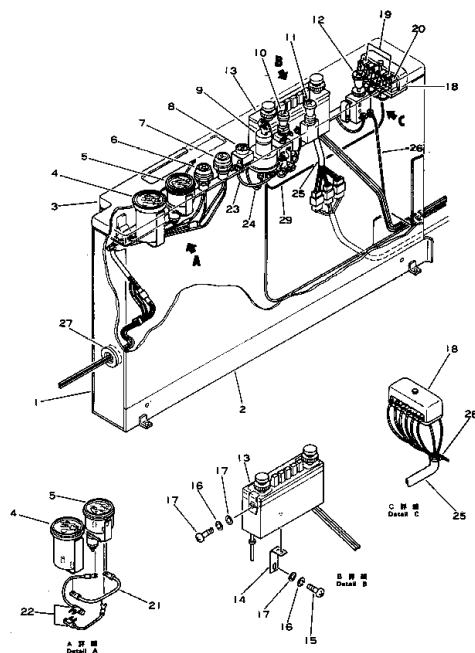
インスツルメント パネル ( 通用機種 ) Fig. 157 INSTRUMENT PANEL (PC60U Serial No. 1001~)
