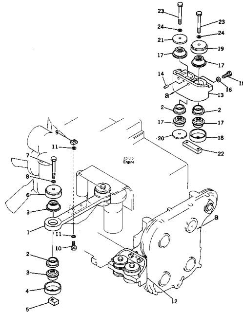
エンジン マウント (PC400 適用機種 Fig. 101 ENGINE MOUNT (Serial No. 10001~10281) (PC400LC Serial No. 10124~10281))
