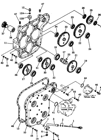
パワー ターク オフ Fig. 105 POWER TAKE OFF (1/2) (PC400 Serial No. 10001~10031)
