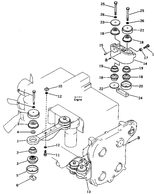
エンジン マウント (PC400 適用機種 Fig. 101A ENGINE MOUNT (Serial No. 10282~) (PC400LC Serial No. 19282~)
