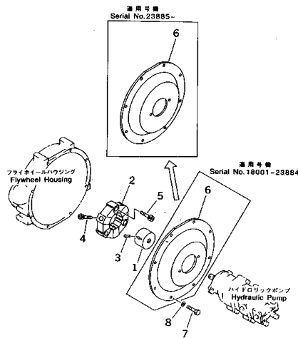
FIG. B0600-01A0 パワーテイクオフ POWER TAKE OFF
