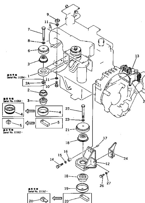
エンジン マウント Fig. 101 ENGINE MOUNT
