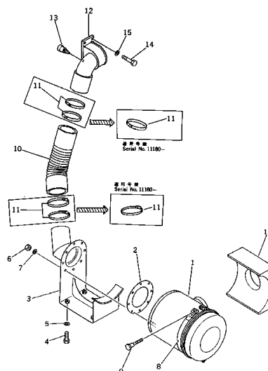
エアークリーナおよびコネクション Fig. 115A AIR CLEANER AND CONNECTION 適用台数 (PC300 Serial No. 11001~) (PC300LC Serial No. 11011~)
