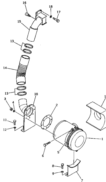
エアークリーナ および コネクション Fig. 115 AIR CLEANER AND CONNECTION (PC300LC Serial No. 11001~11010)
