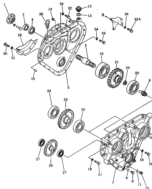
パワー テーク オフ Fig. 105 POWER TAKE OFF
