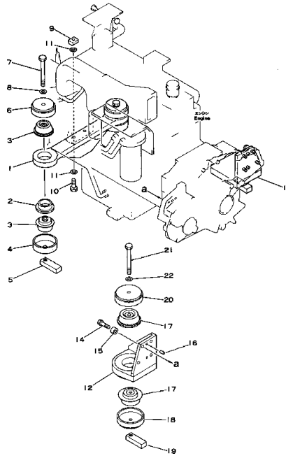
エンジンマウント Fig. 101 ENGINE MOUNT
