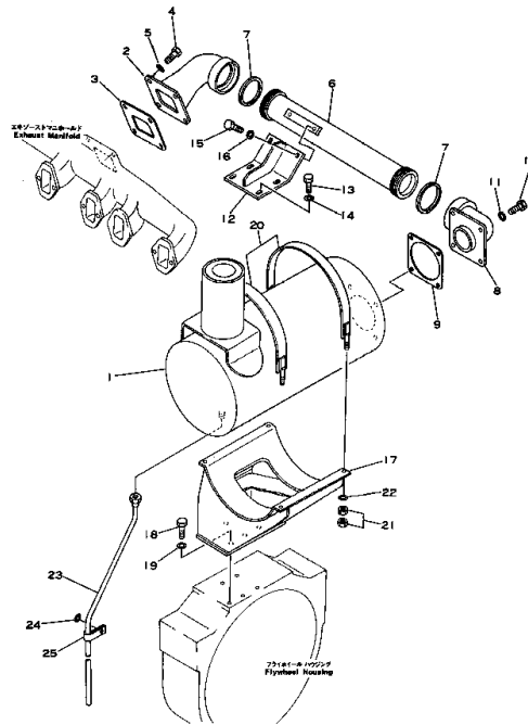
マフラー および コネクション Fig. 111 MUFFLER AND CONNECTION
