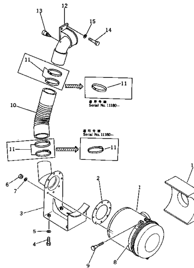
エアークリーナおよびコネクション Fig. 115A AIR CLEANER AND CONNECTION 適用台数 (PC300 Serial No. 11001~) (PC300LC Serial No. 11011~)
